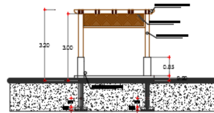
ALZADO PERGOLADO
