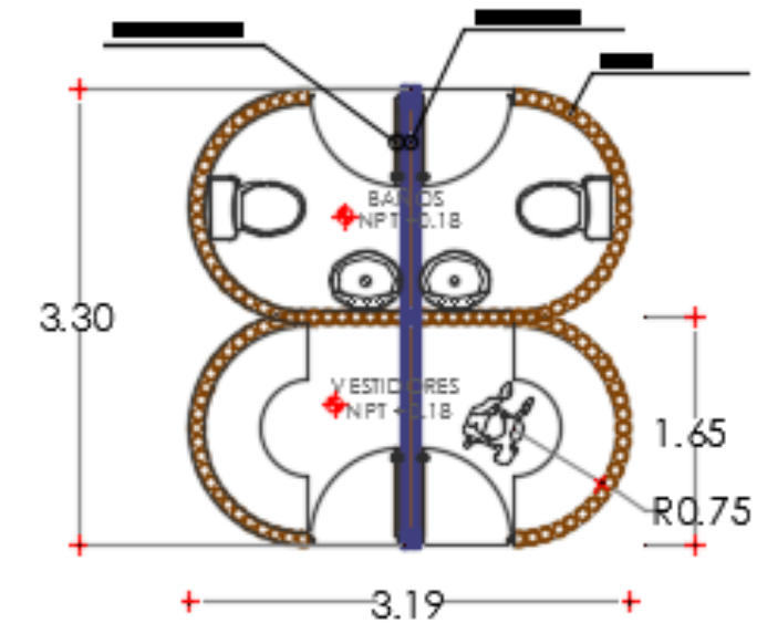
PLANTA VESTIDORES / BAÑOS
