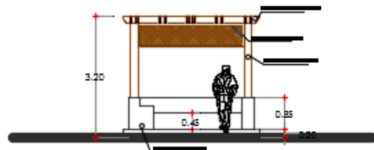
ALZADO PERGOLADO
