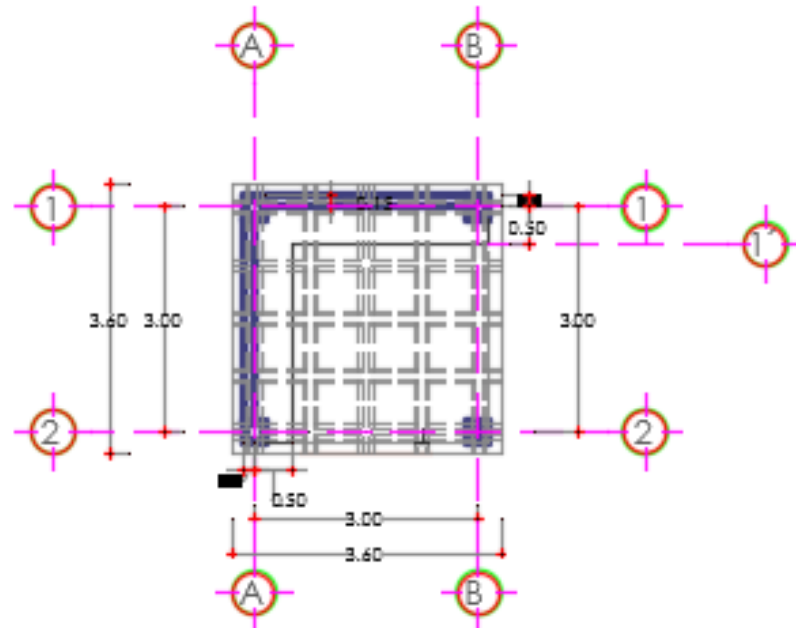
PLANTA PERGOLADO TEMAZCAL
