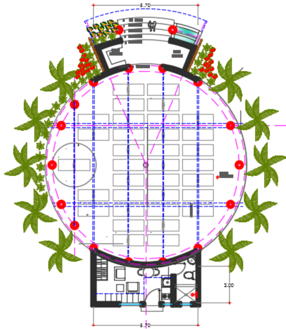
PLANTA ARQUITECTÓNICA CENTRO DE YOGA
