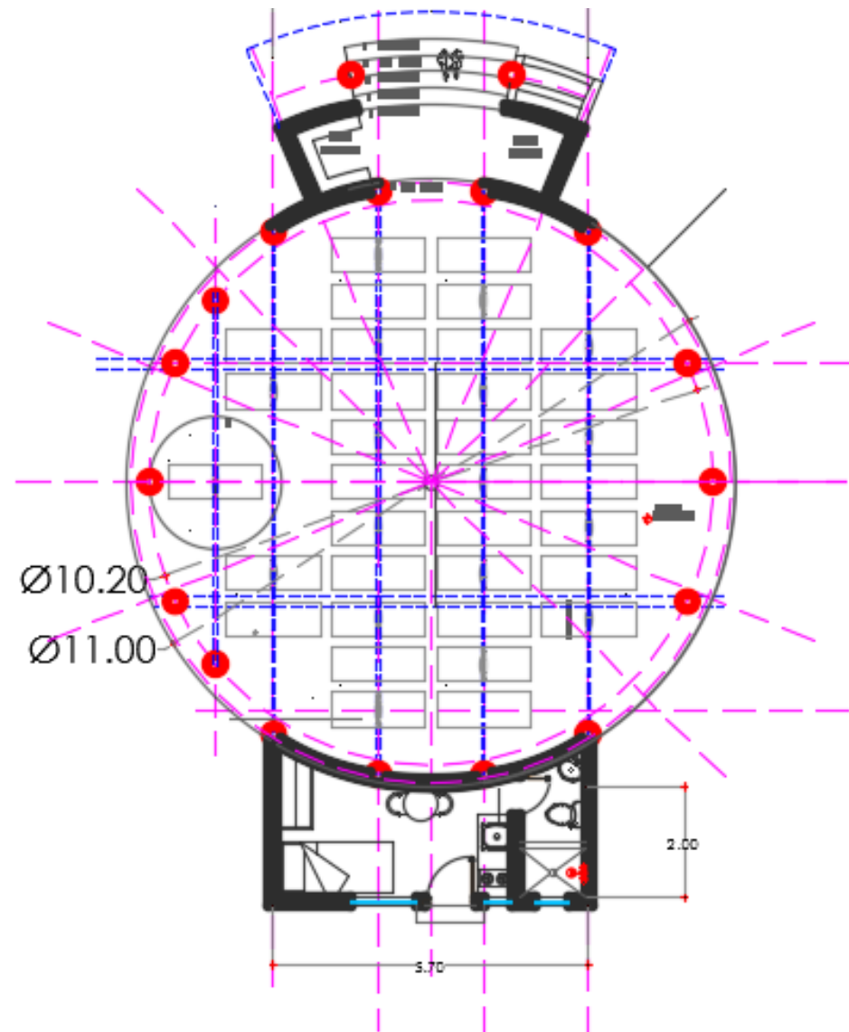
PLANTA ARQUITECTÓNICA CENTRO DE YOGA
