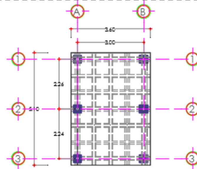
PLANTA PERGOLADO PALAFITO
